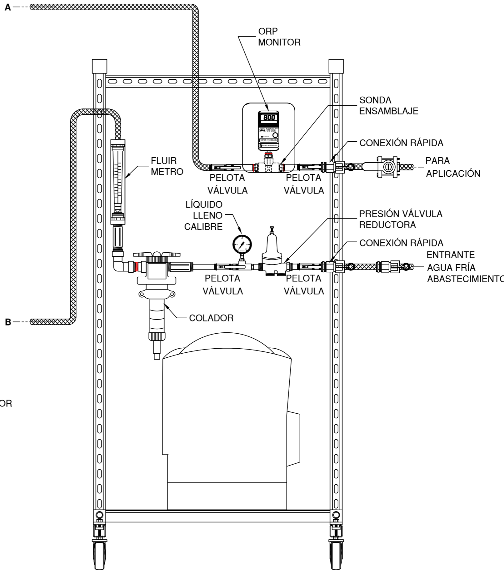
VISTA TRASERA
