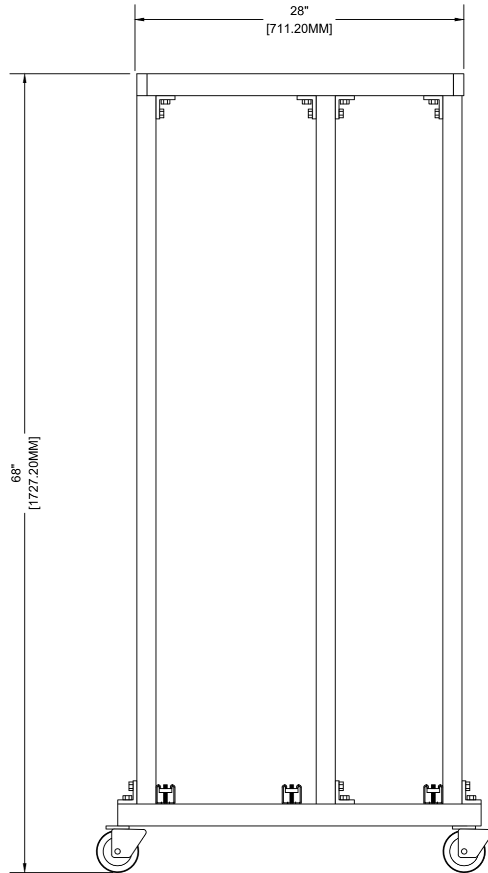
VISTA LATERAL
